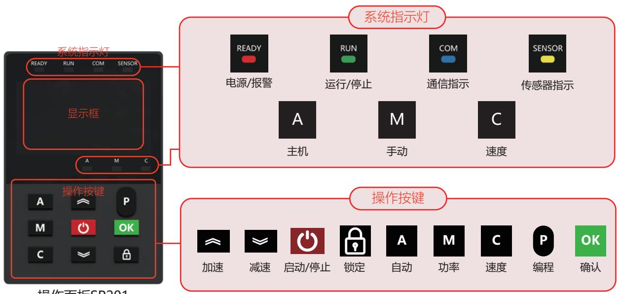
操作面板SP201
