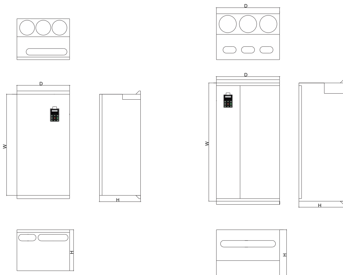
外形DIM: R503 R505 R506
